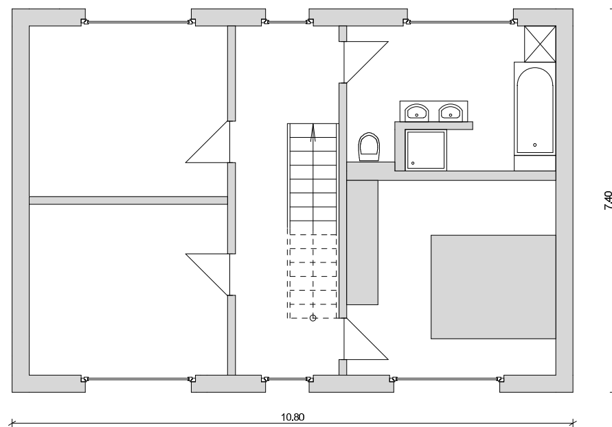
Grundriss OG
