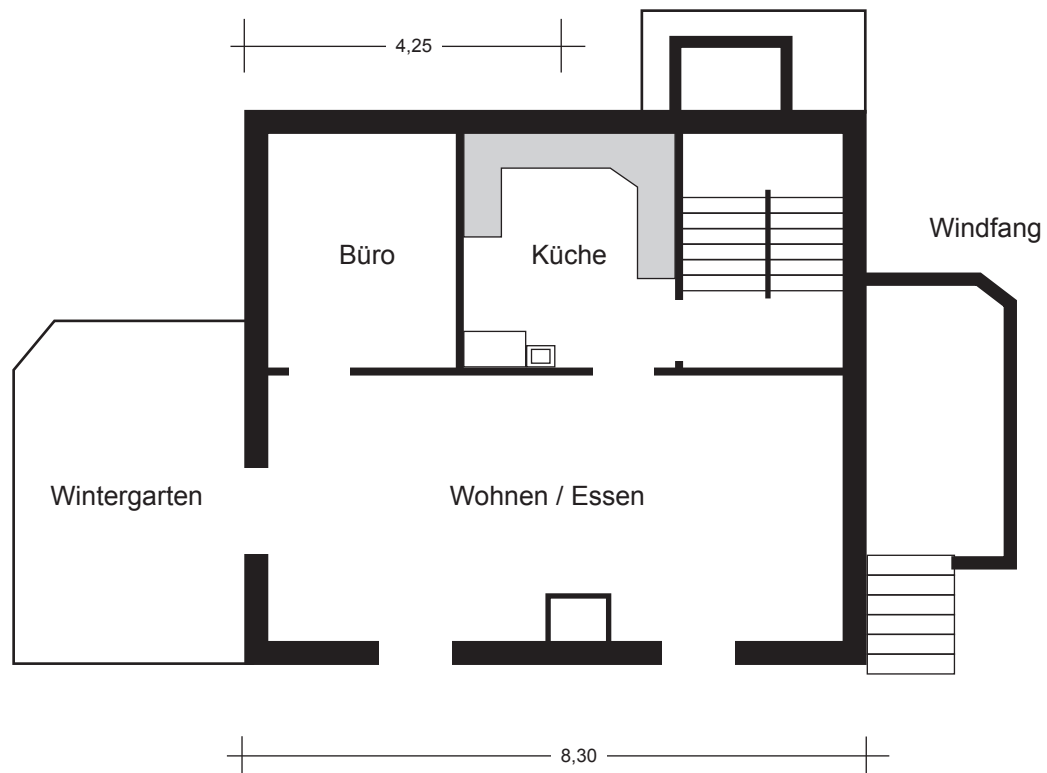
Erdgeschoss 1:100
